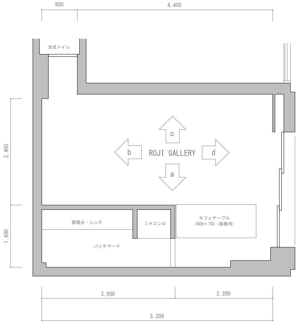
平面図 S = 1 / 50
